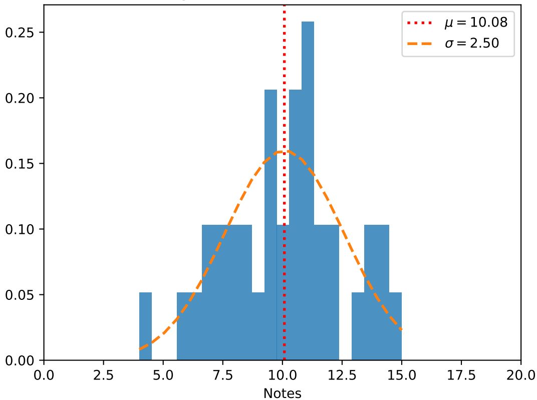
Histogramme des notes du DS n°05
